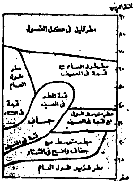
توزيع نظري على سطح الأرض
